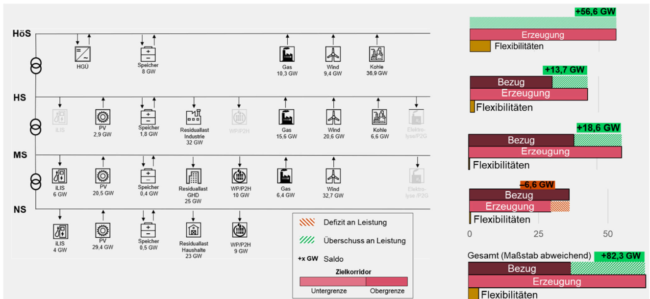
Abbildung 13: Das Stromnetz und seine Stellregler im Status quo
